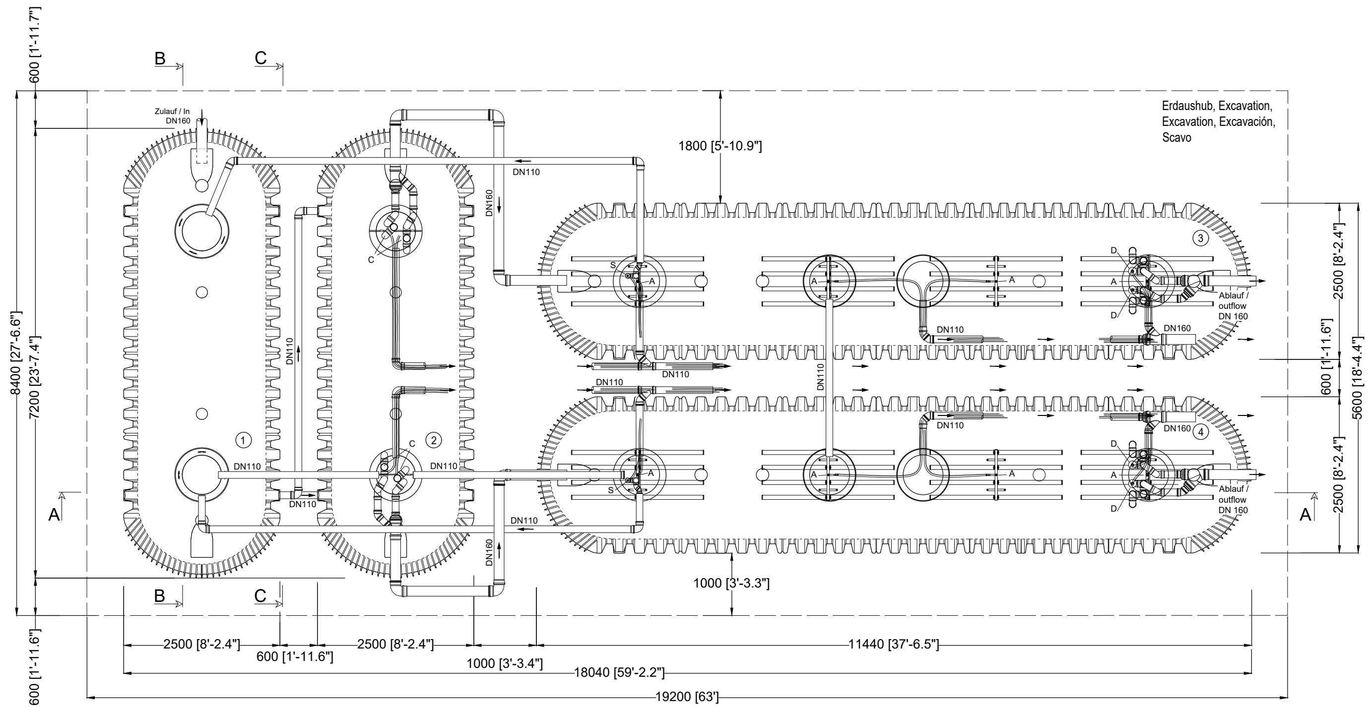
Vorklärung / Schlamm Speicher Pre-treatment / Sludge storage
